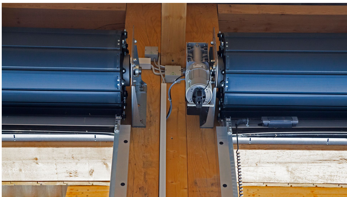
Industrie Rolltor Detail Lager und Motor
